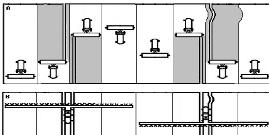
Figure 4. Confection de voies d'accès en deux passage.
