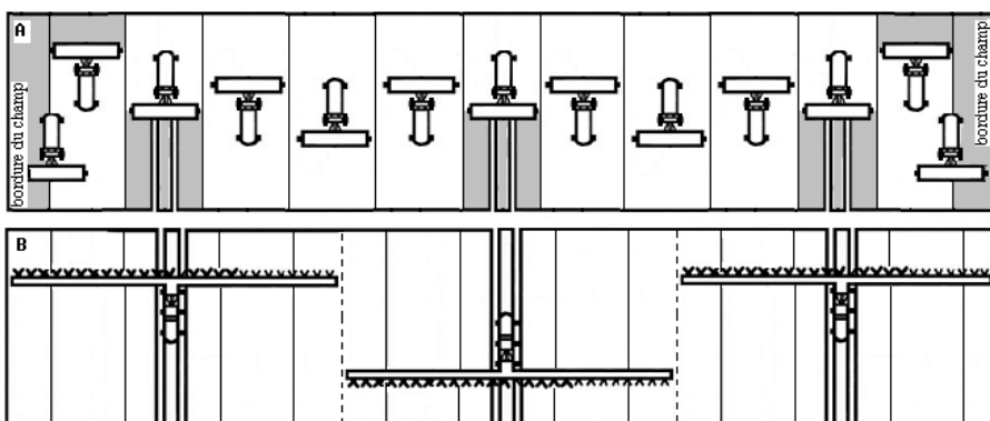
Figure 3. Confection de voies d'accès lorsque le ratio largeurs semoir / équipement de traitement est pair.
